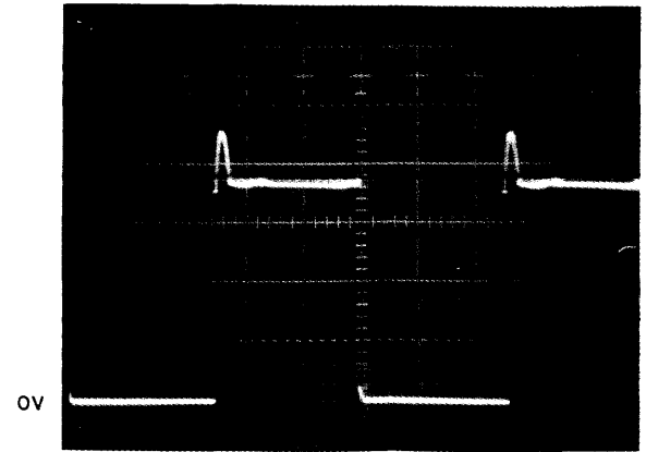
Q11 Collector Voltage
