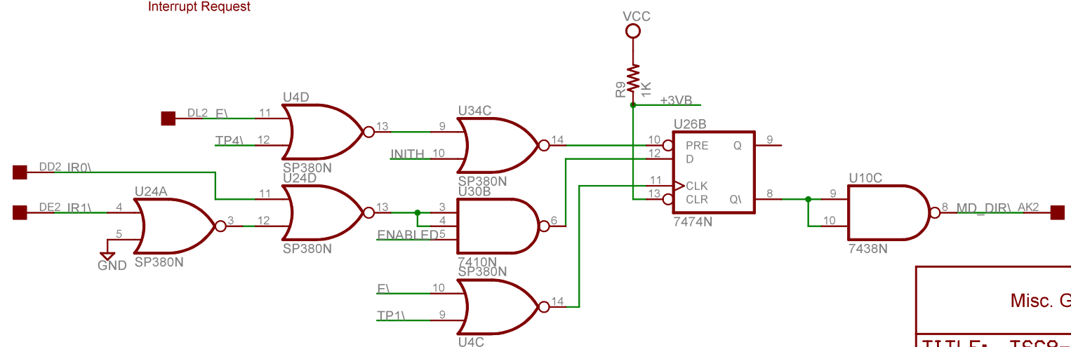
MD DIR
