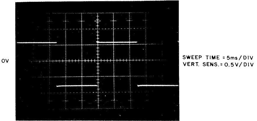
Q11 Emitter to Base Voltage
